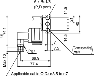
DIN terminal: D
