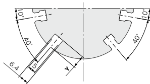
オートスイッチ取付用溝位置
