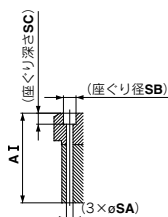
SD-SD断面
