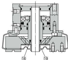
φ32~φ80 開状態
