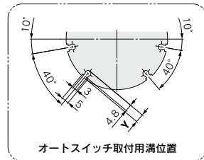
オートスイッチ取付用溝位置
