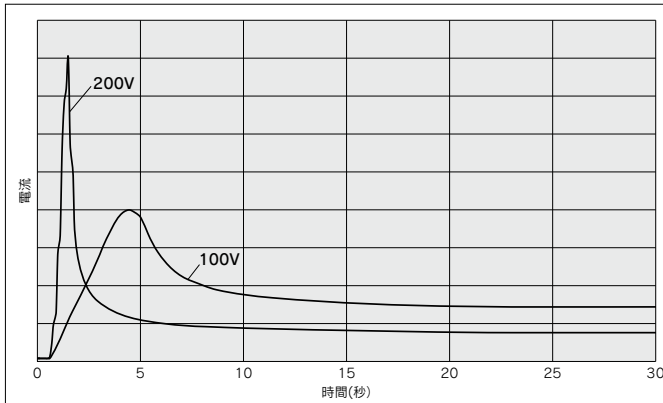
突入電流の流れる時間(目安)
