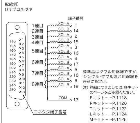
配線仕様特殊[-K]
