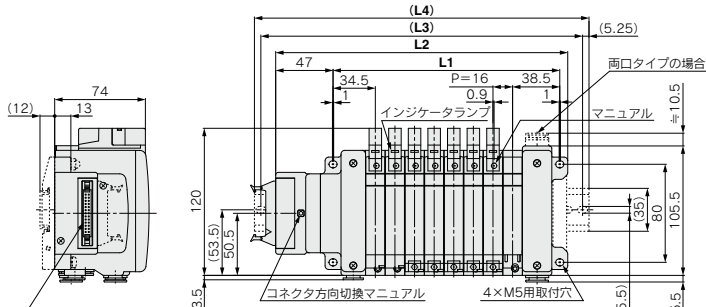
適用コネクタ:フラットケーブル用コネクタ(26P) (MIL-C-83503準拠品)
