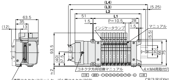
適用コネクタ:フラットケーブル用コネクタ(26P) (MIL-C-83503準拠品)
