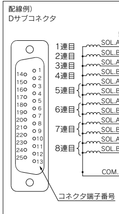
配線仕様特殊[-K]
