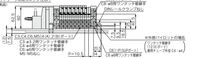
適用コネクタ:フラットケーブル用コネクタ(26P) (MIL-C-83503準拠品)
