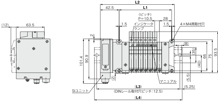
D側 (逆数) ①-②-③-④-⑤-⑥-⑦-⑧ U側
