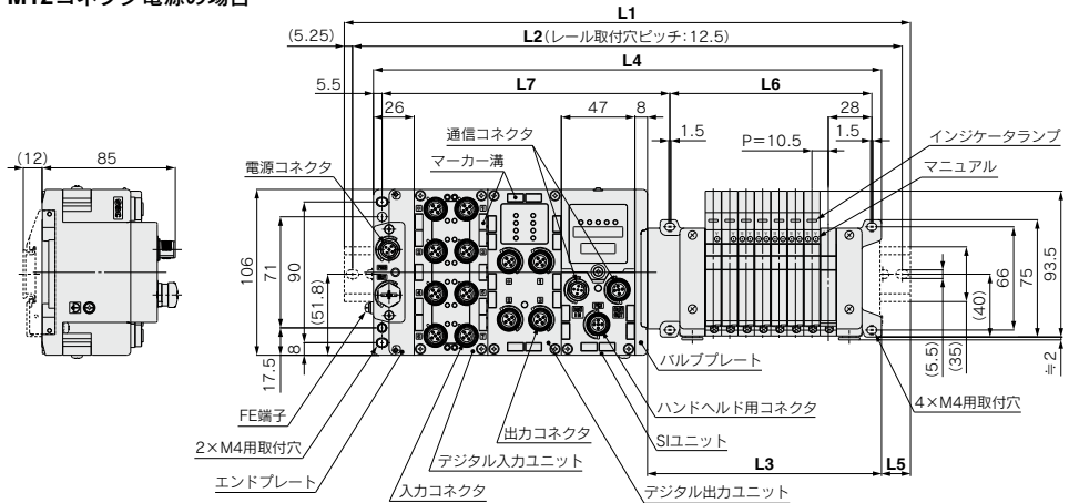
D側 (選数) ①②③④⑤⑥⑦⑧⑨⑩ U側
