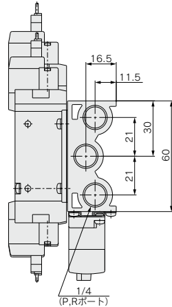
ワンタッチ管継手内蔵形の場合
