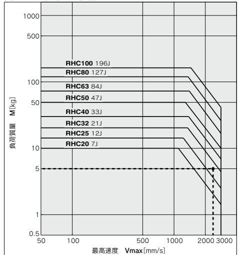
図1-2 垂直駆動 供給圧力0.5MPa
