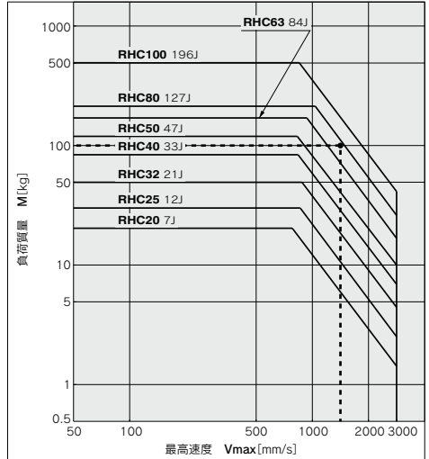
図1-1 水平駆動 供給圧力0.5MPa
