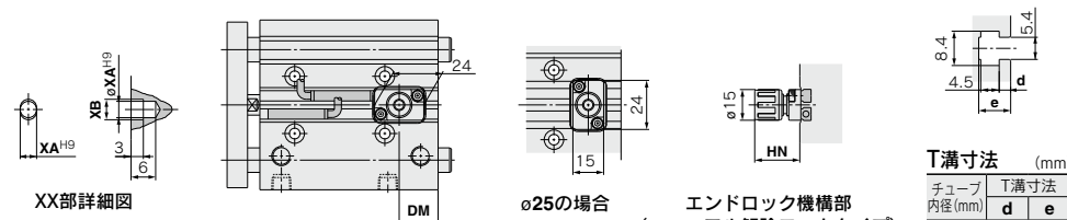
ロッド側ロック付
