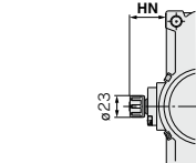
エンドロック機構部 (マニュアル解除ロックタイプ)
