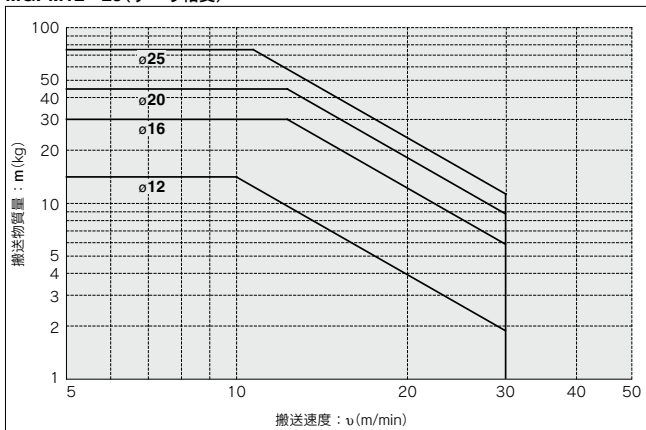
MGPM12~25(すべり軸受)
