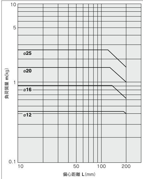
9 30ストローク以下 V=400mm/s
