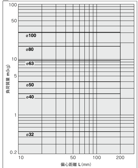
12 50ストロークを超える V=400mm/s
