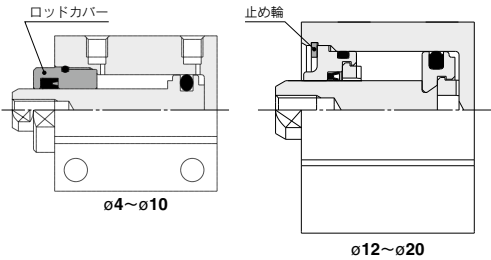
ø12~ø20
