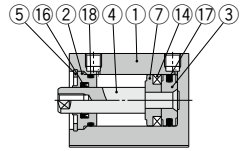
オートスイッチ付(磁石内蔵) ø12, ø16
