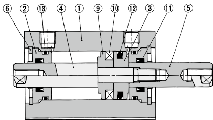
φ12、φ16
