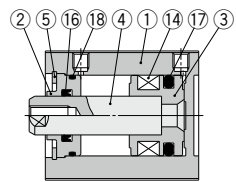
ø20, ø25
