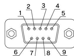
警報出力コネクタ D-sub 9ピン(ピンタイプ)
