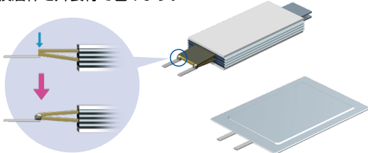
TAB溶着
