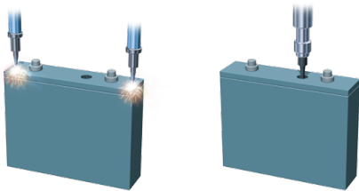
セル蓋溶接
